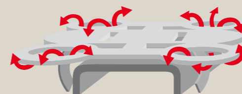
Drukverdeling door flexibele schotelveren
