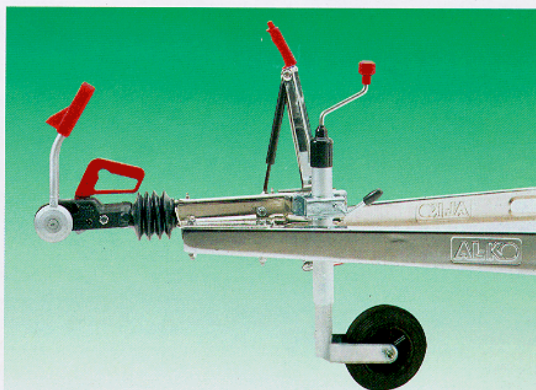
Deze koppeling is het belevings: het veiligheidskoppelingssysteem AKS 2000 (standaard bij Diamant en Joker, tot type 496 AKS 1300 ) temper bij hoge snelheid voelbaar de slingerbewegingen – en zorgt daarmee voor maximale rijveiligheid.
